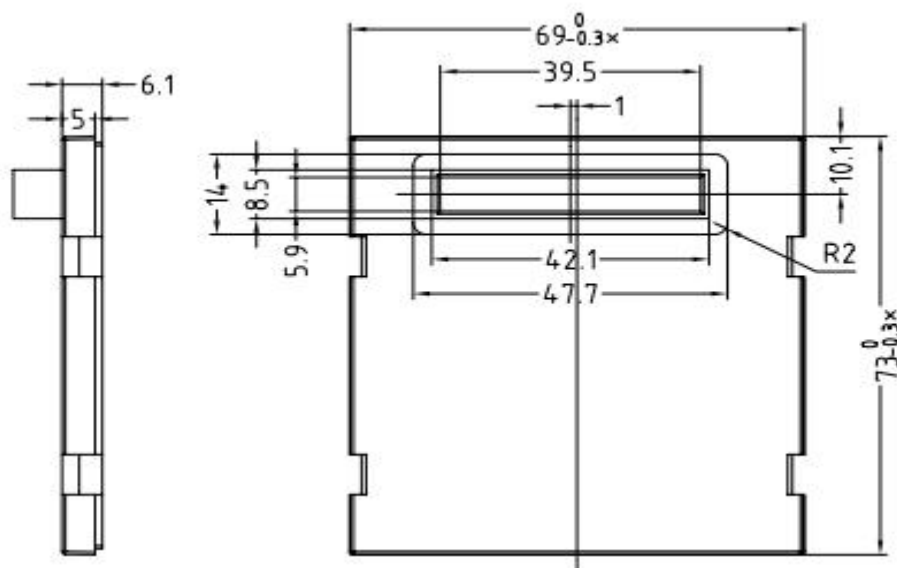
图5 正面尺寸
